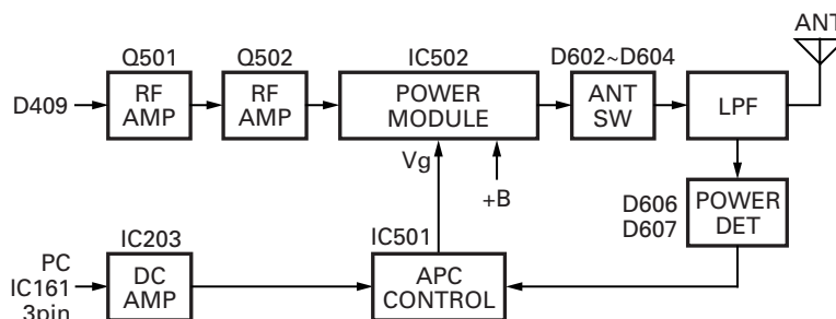
Fig. 9 APC circuit / 图9 自动功率控制电路
